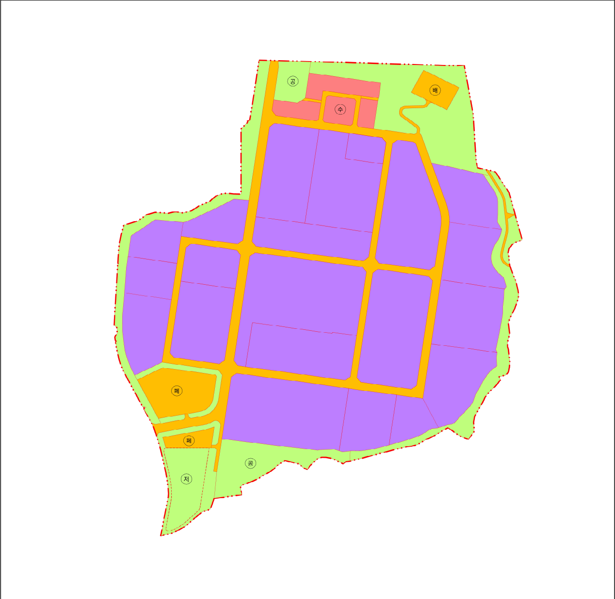
괴산 첨단산업단지계획 변경 용도별 구역계획 평면도
